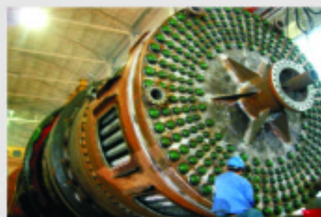
焦化设备
